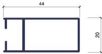
MARCO DE HOJA LATERAL- 2010
