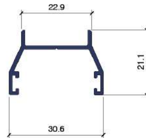
PERFIL ADAPTADOR DE HOJA- 2008
