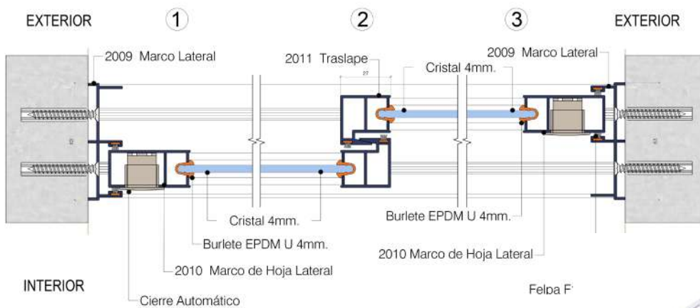
CORTE HORIZONTAL
