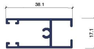
MARCO DE HOJA SUPERIOR- 2004
