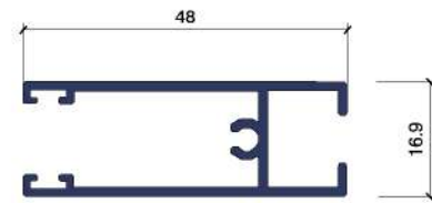
MARCO DE HOJA INFERIOR- 2005
