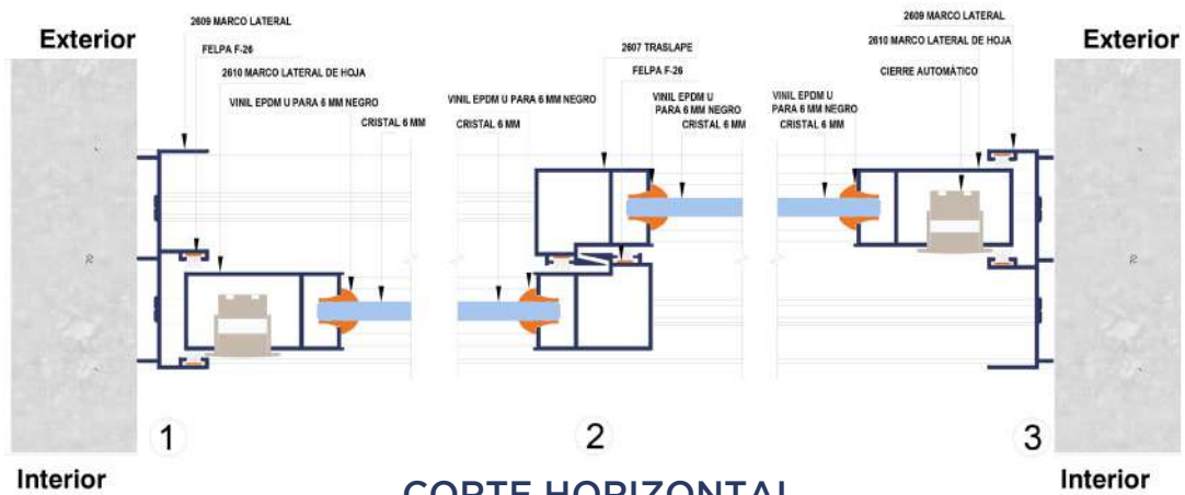
CORTE HORIZONTAL
