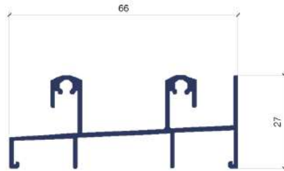
MARCO INFERIOR 2502
