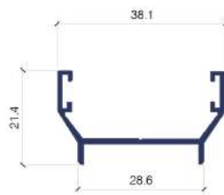
PERFIL ADAPTADOR 2508
