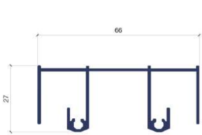
MARCO SUPERIOR 2501
