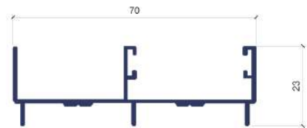
MARCO LATERAL 2509
