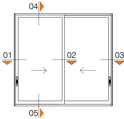
ELEVACION
