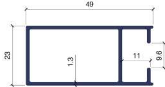
VL4206 MARCO DE HOJA LATERAL
