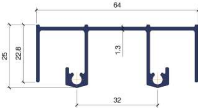
VL4201 MARCO SUPERIOR
