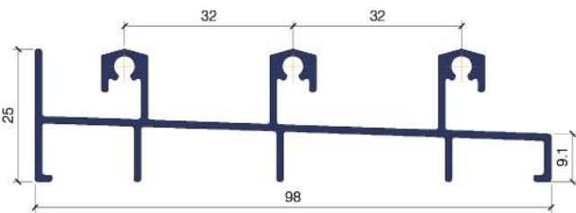
VL 4216 MARCO INFERIOR TRIPLE
