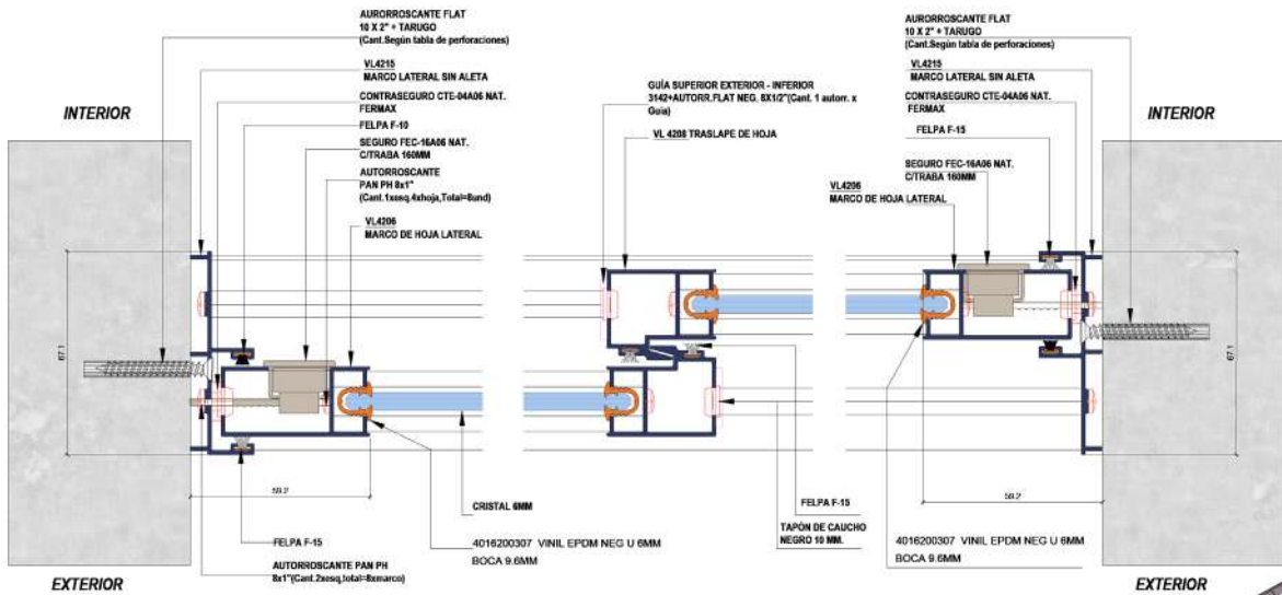
CORTE HORIZONTAL
