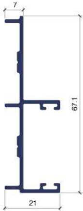
VL4215 MARCO LATERAL SIN ALETA
