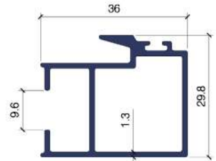
VL 4208 TRASLAPE DE HOJA
