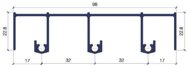
VL 4217 MARCO SUPERIOR TRIPLE
