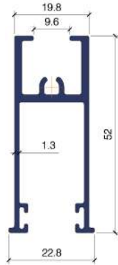
VL 4210 MARCO DE HOJA INFERIOR REFORZADO
