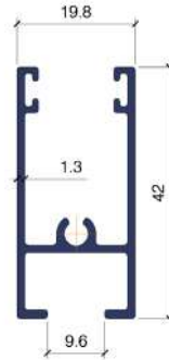
VL 4209 MARCO DE HOJA SUPERIOR
