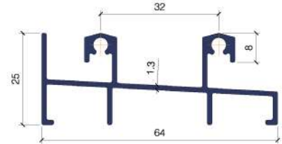
VL4202 MARCO INFERIOR
