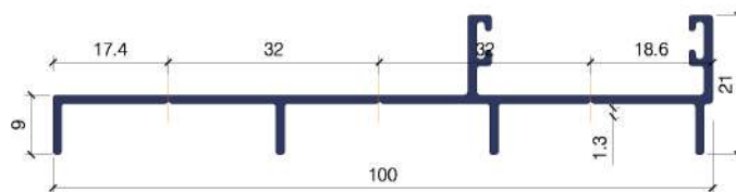
VL 4218 MARCO LATERAL TRIPLE
