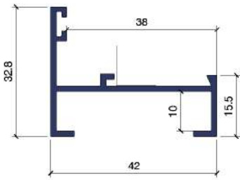
3601 MARCO PROYECTANTE
