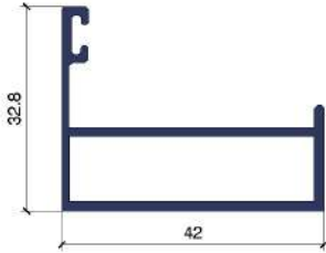
3606 MARCO
