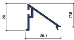
3604 JUNQUILLO
