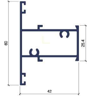
3603 TRAVESAÑO
