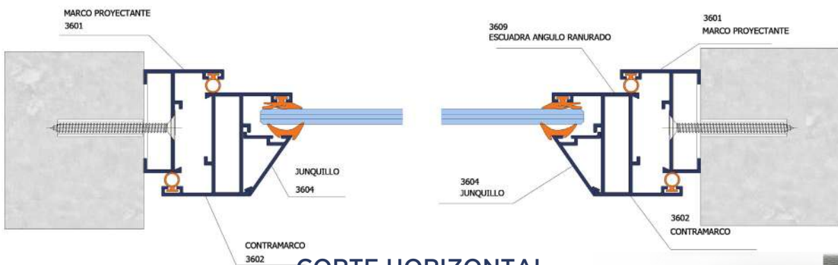
CORTE HORIZONTAL
