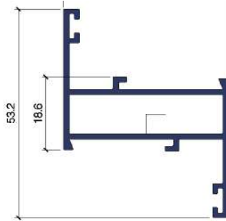
3602 CONTRAMARCO
